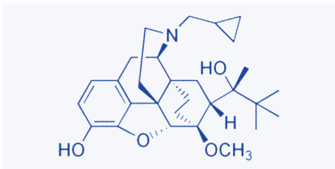
Estructura química de Buprenorfina. Imagen tomada de http://es.wikipedia.org/wiki/Archivo:Buprenorphine_structure.png
